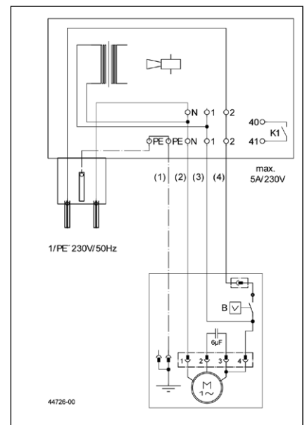
Schakelbeeld
