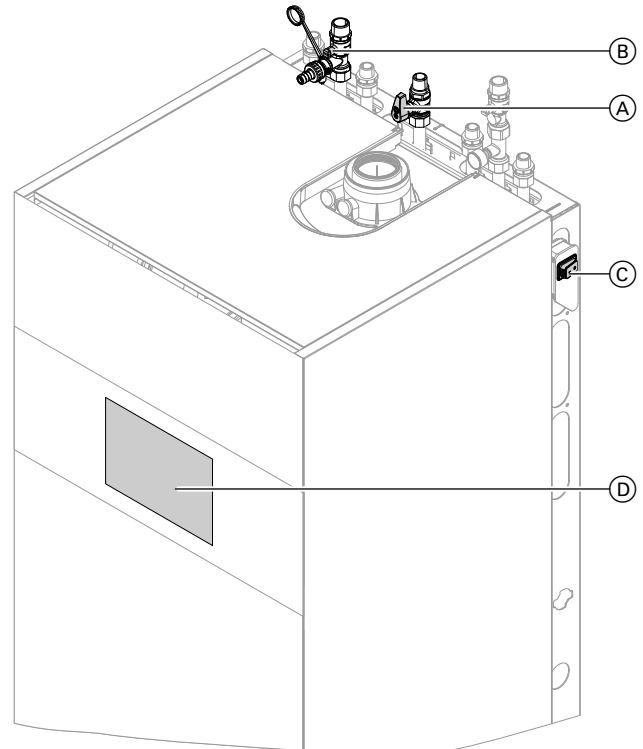
Abb. 5 Beispiel mit Anschlüssen nach oben
