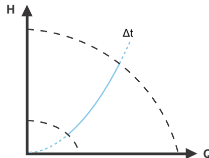
Abb. 39 Differenztemperatur
