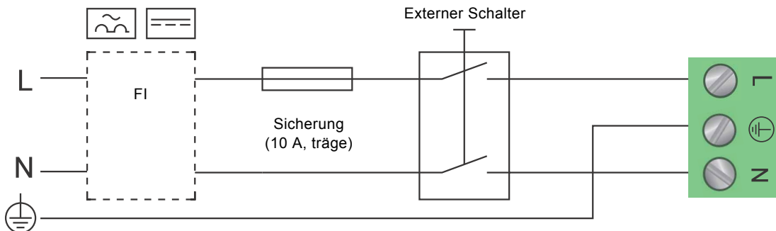
Abb. 20 Beispiel für einen typischen Netzanschluss, 1 x 230 V ± 10 %, 50/60 Hz, PE
