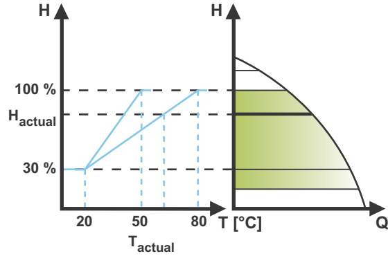
Abb. 47 Temperaturführung
