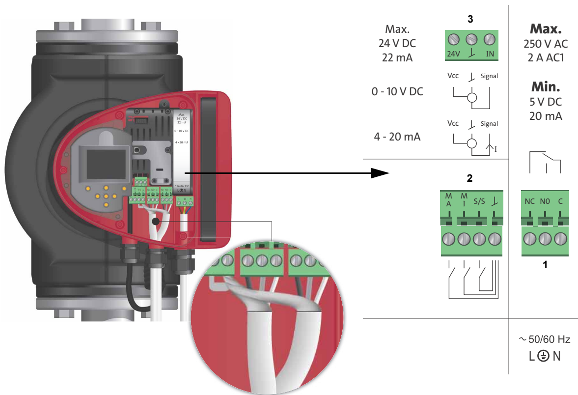
Abb. 22 Schaltplan bei mit Klemmen angeschlossenen Ausführungen
