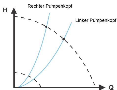
Abb. 51 Hydraulischer Unterschied zwischen den beiden Köpfen
