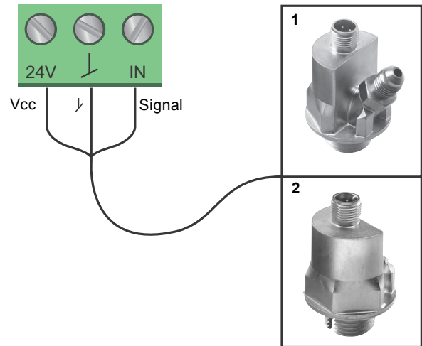
Abb. 28 Beispiele für externe Sensoren
