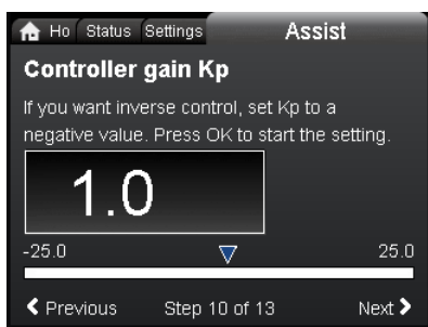
Abb. 43 Regler, Verstärkung K_p
