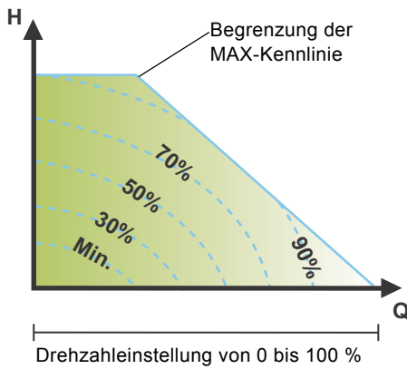
Abb. 42 Begrenzung der MAX-Kennlinie durch eine Leistungs- und Druckbegrenzung
