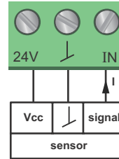
Abb. 27 Analogeingang für den Anschluss eines externen Sensors, 4-20 mA
