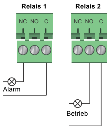
Abb. 24 Relaisausgang
