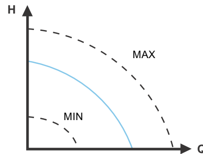
Abb. 33 MIN- und MAX-Kennlinie
