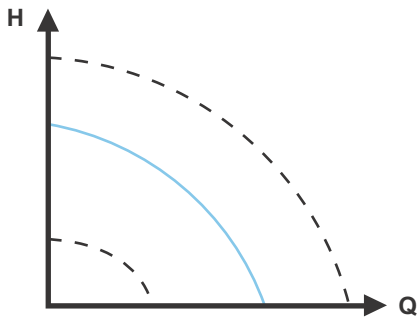
Abb. 41 Konstante Kennlinie
