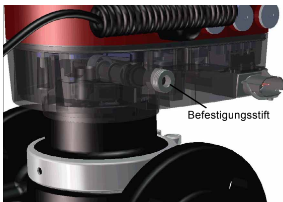
Abb. 13 Befestigungsstift für mit Stecker angeschlossene Ausführungen
