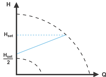
Abb. 36 Proportionaldruck
