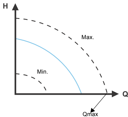
Abb. 49 Q_{max}
