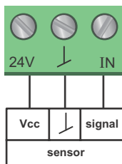
Abb. 26 Analogeingang für den Anschluss eines externen Sensors, 0-10 V
