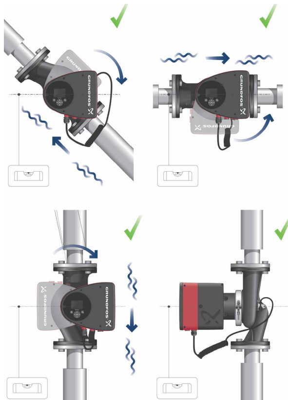
Abb. 15 Pumpe mit horizontal ausgerichteter Elektronikeinheit
