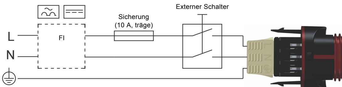
Abb. 21 Beispiel für einen Netzanschluss mit ALPHA-Stecker, 1 x 230 V ± 10 %, 50/60 Hz, PE
