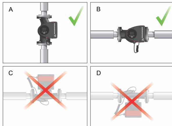
Abb. 14 Pumpe mit horizontal ausgerichteter Motorwelle
