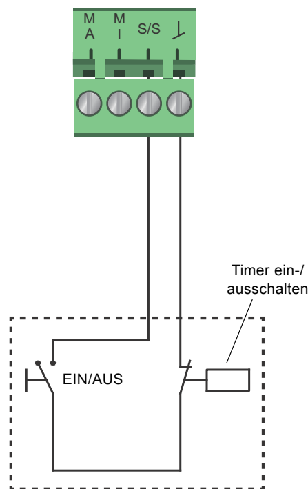
Abb. 25 Digitaleingang
