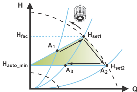
Abb. 34 AUTO_{ADAPT}
