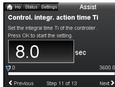
Abb. 44 Regler, Integrationszeit T_i
