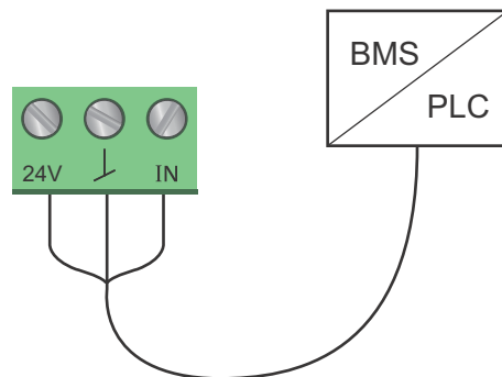
Abb. 29 Beispiel für ein externes Steuersignal für die Regelung über eine GLT/SPS
