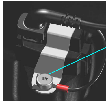
Abb. 53 Masseverbindung des Sensors
