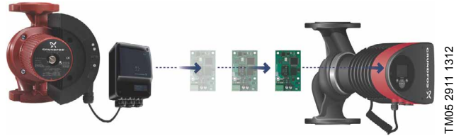
Abb. 55 Weiterverwenden eines CIM-Moduls
