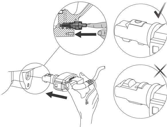
Abb. 52 Richtige Sensoranordnung
