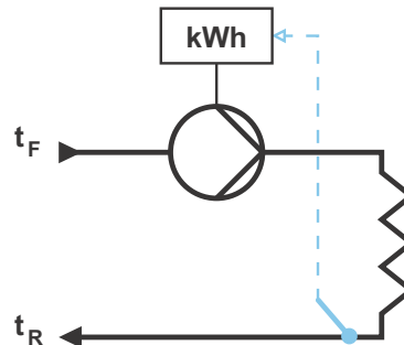
Abb. 48 MAGNA3 mit integriertem Wärmemengenzähler
