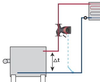
Abb. 40 Differenztemperatur
