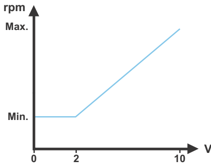
Abb. 46 Externe Sollwertfunktion, 0 bis 10 V
